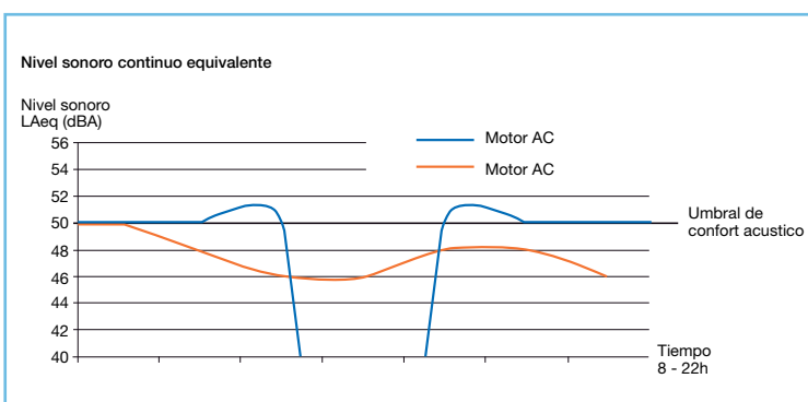
Grafica comparativa Nivel sonoro
