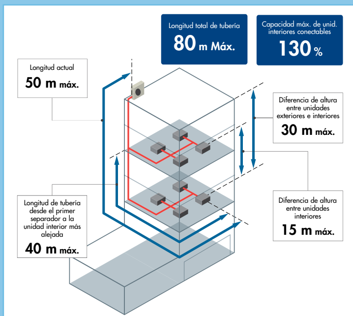
Distancias frigoríficas.
