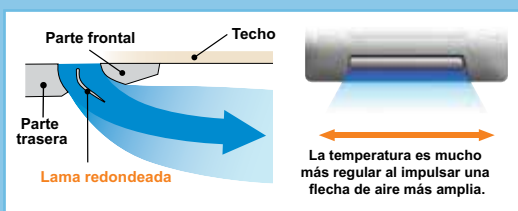
Nuevo diseño de lama.
