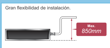
Bomba de condensados incluida
